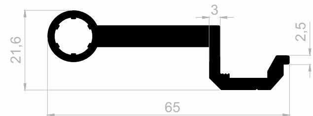
J 1623 SCHARNIERPROFILE GEWICHT : 1,019 kg/m
