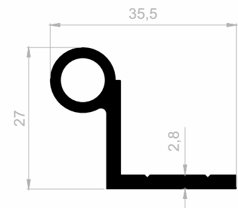
J 1141 SCHARNIERPROFILE GEWICHT : 0,494 kg/m
