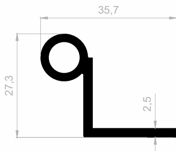
J 1943 SCHARNIERPROFILE GEWICHT : 0,477 kg/m
