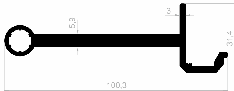
J 1619 SCHARNIERPROFILE GEWICHT : 1,696 kg/m
