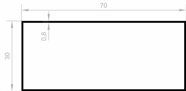
J 2242 LINEAL PROFILE (LUXUS SERIE) GEWICHT : 0,425 kg/m
