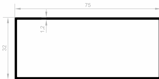
J 6167 LINEAL PROFILE (ECONOMIC SERIE) GEWICHT : 0,680 kg/m
