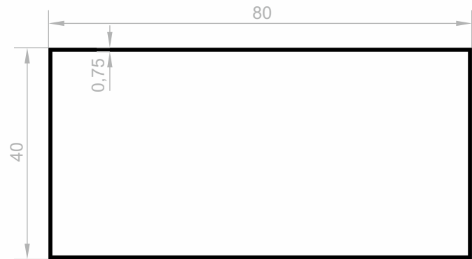
J 1559 LINEAL PROFILE (LUXUS SERIE) GEWICHT : 0,482 kg/m
