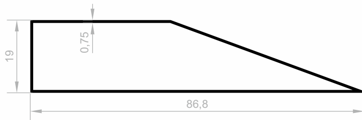
J 3746 LINEAL PROFILE (LUXUS SERIE) GEWICHT : 0,390 kg/m
