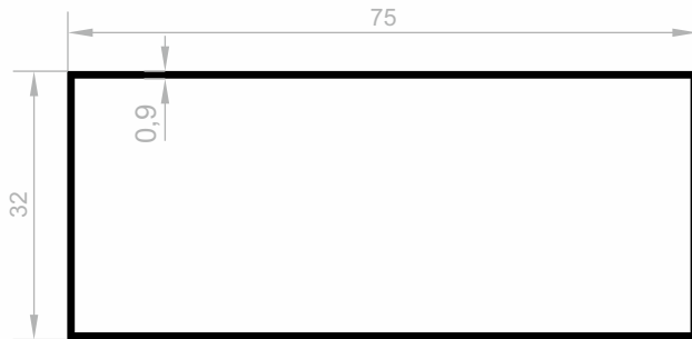
J 1025 LINEAL PROFILE (LUXUS SERIE) GEWICHT : 0,512 kg/m
