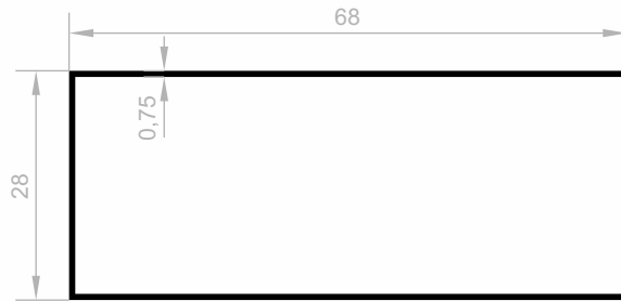
J 3747 LINEAL PROFILE (LUXUS SERIE) GEWICHT : 0,390 kg/m
