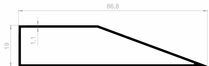
NEU J 8501 LINEAL PROFILE (LUXUS SERIE) GEWICHT : 0,566 kg/m
