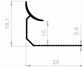
JF 3515 FLIESEN PROFILE GEWICHT : 0,081 kg/m
