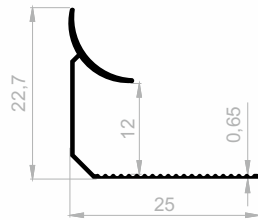
JF 2166 FLIESEN PROFILE GEWICHT : 0,095 kg/m
