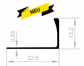
JF 8448 FLIESEN PROFILE GEWICHT : 0,078 kg/m
