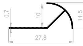
JF 8226 FLIESEN PROFILE GEWICHT : 0,081 kg/m
