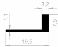
JF 2100 FLIESEN PROFILE GEWICHT : 0,117 kg/m
