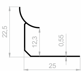
JF 8172 FLIESEN PROFILE GEWICHT : 0,079 kg/m
