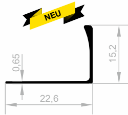
JF 8449 FLIESEN PROFILE GEWICHT : 0,083 kg/m
