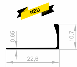
JF 8447 FLIESEN PROFILE GEWICHT : 0,073 kg/m
