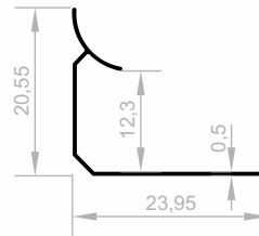
JF 6221 FLIESEN PROFILE GEWICHT : 0,065 kg/m
