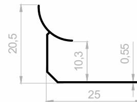
JF 3425 FLIESEN PROFILE GEWICHT : 0,109 kg/m
