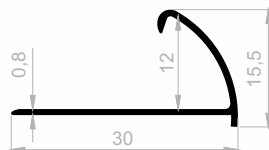
JF 1978 FLIESEN PROFILE GEWICHT : 0,117 kg/m
