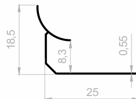
JF 8173 FLIESEN PROFILE GEWICHT : 0,073 kg/m
