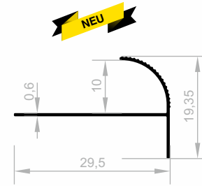
JF 8259 FLIESEN PROFILE GEWICHT : 0,089 kg/m
