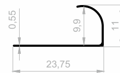
JF 6068 FLIESEN PROFILE GEWICHT : 0,057 kg/m
