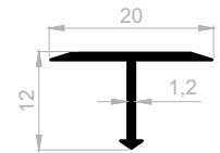
JF 3940 FLIESEN PROFILE GEWICHT : 0,095 kg/m
