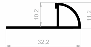
JF 3190 FLIESEN PROFILE GEWICHT : 0,163 kg/m
