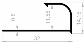
JF 2971 FLIESEN PROFILE GEWICHT : 0,121 kg/m
