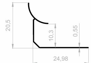
JF 3426 FLIESEN PROFILE GEWICHT : 0,119 kg/m
