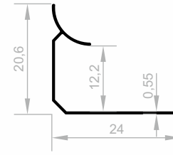
JF 8445 FLIESEN PROFILE GEWICHT : 0,074 kg/m
