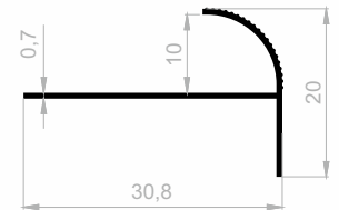
JF 1583 FLIESEN PROFILE GEWICHT : 0,108 kg/m
