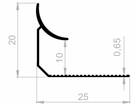
JF 2141 FLIESEN PROFILE GEWICHT : 0,089 kg/m
