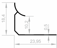
JF 6189 FLIESEN PROFILE GEWICHT : 0,063 kg/m
