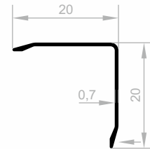
JF 8468 FLIESEN PROFILE GEWICHT : 0,076 kg/m
