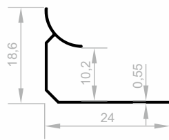
JF 8436 FLIESEN PROFILE GEWICHT : 0,071 kg/m
