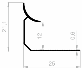
JF 3516 FLIESEN PROFILE GEWICHT : 0,085 kg/m
