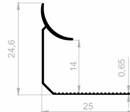
JF 2282 FLIESEN PROFILE GEWICHT : 0,098 kg/m
