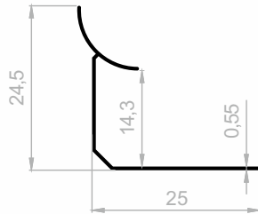
JF 8171 FLIESEN PROFILE GEWICHT : 0,081 kg/m
