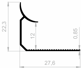
JF 3392 FLIESEN PROFILE GEWICHT : 0,114 kg/m
