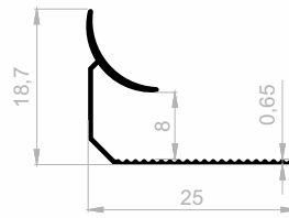
JF 2687 FLIESEN PROFILE GEWICHT : 0,087 kg/m
