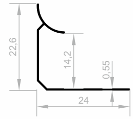
JF 3393 FLIESEN PROFILE GEWICHT : 0,108 kg/m
