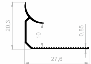
JF 3393 FLIESEN PROFILE GEWICHT : 0,108 kg/m
