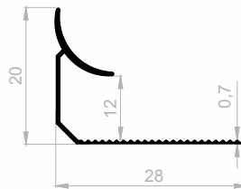
JF 1582 FLIESEN PROFILE GEWICHT : 0,103 kg/m
