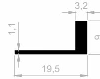
JF 1026 FLIESEN PROFILE GEWICHT : 0,127 kg/m
