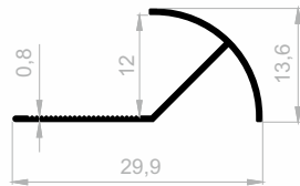
JF 2206 FLIESEN PROFILE GEWICHT : 0,106 kg/m
