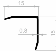
JF 8231 FLIESEN PROFILE GEWICHT : 0,062 kg/m
