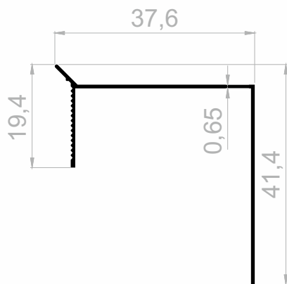
J 1935 FENSTERBÄNKE GEWICHT : 0,173 kg/m
