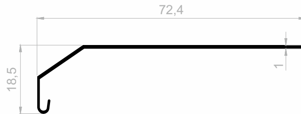
J 2114 FENSTERBÄNKE GEWICHT : 0,230 kg/m
