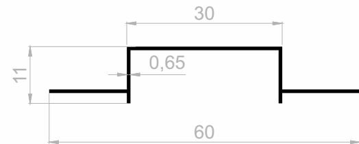
J 1939 FENSTERBÄNKE GEWICHT : 0,152 kg/m
