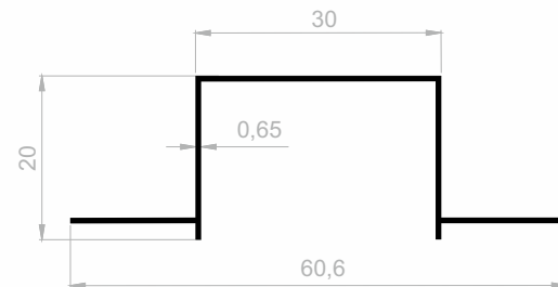
J 1937 FENSTERBÄNKE GEWICHT : 0,187 kg/m
