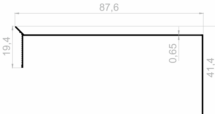
J 1934 FENSTERBÄNKE GEWICHT : 0,268 kg/m
