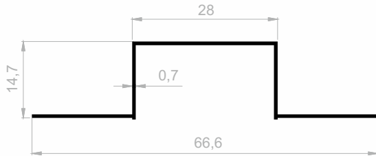
J 1938 FENSTERBÄNKE GEWICHT : 0,168 kg/m
