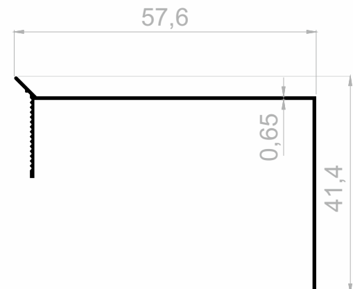
J 1928 FENSTERBÄNKE GEWICHT : 0,211 kg/m
