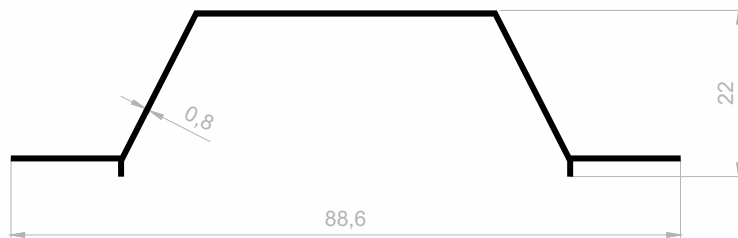
J 2101 FENSTERBÄNKE GEWICHT : 0,252 kg/m
