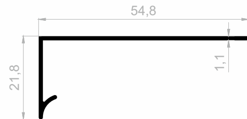
J 2200 FENSTERBÄNKE GEWICHT : 0,238 kg/m
