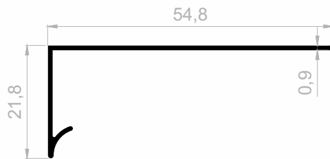
J 2465 FENSTERBÄNKE GEWICHT : 0,198 kg/m
