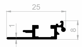
J 1204 DISPLAY PROFILE GEWICHT : 0,300 kg/m
