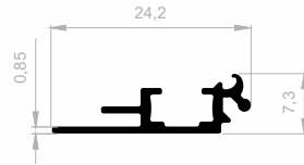
J 19126 DISPLAY PROFILE GEWICHT : 0,122 kg/m
