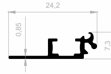
J 8215 DISPLAY PROFILE GEWICHT : 0,111 kg/m
