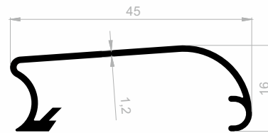
J 1183 DISPLAY PROFILE GEWICHT : 0,273 kg/m
