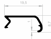
J 1199 DISPLAY PROFILE GEWICHT : 0,089 kg/m
