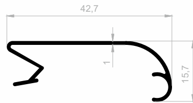
J 1160 DISPLAY PROFILE GEWICHT : 0,217 kg/m
