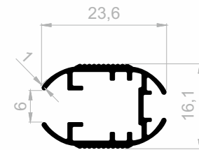
J 1613 DISPLAY PROFILE GEWICHT : 0,245 kg/m
