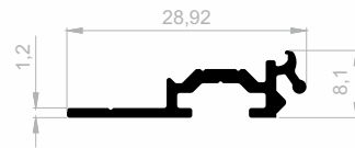
J 19120 DISPLAY PROFILE GEWICHT : 0,146 kg/m
