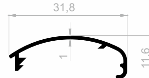
J 1182 DISPLAY PROFILE GEWICHT : 0,138 kg/m
