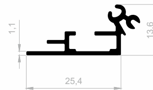
J 19123 DISPLAY PROFILE GEWICHT : 0,222 kg/m
