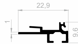
J 1162 DISPLAY PROFILE GEWICHT : 0,688 kg/m
