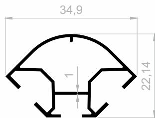
J 1963 DISPLAY PROFILE GEWICHT : 0,287 kg/m
