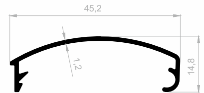
J 1579 DISPLAY PROFILE GEWICHT : 0,233 kg/m
