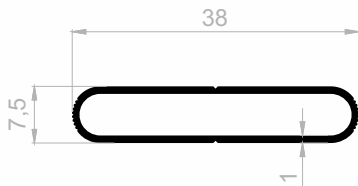
J 1202 DISPLAY PROFILE GEWICHT : 0,216 kg/m
