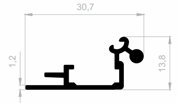
J 1179 DISPLAY PROFILE GEWICHT : 0,224 kg/m
