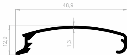
J 1181 DISPLAY PROFILE GEWICHT : 0,275 kg/m
