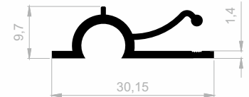
J 1173 DISPLAY PROFILE GEWICHT : 0,205 kg/m
