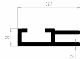
J 1187 DISPLAY PROFILE GEWICHT : 0,348 kg/m
