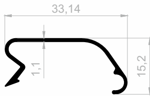
J 19125 DISPLAY PROFILE GEWICHT : 0,157 kg/m
