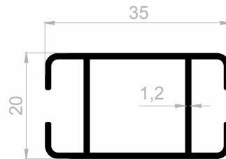
J 1185 DISPLAY PROFILE GEWICHT : 0,405 kg/m
