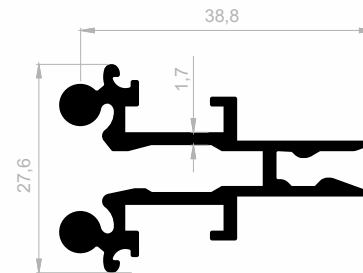
J 1162 DISPLAY PROFILE GEWICHT : 0,688 kg/m
