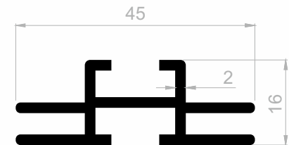
J 1186 DISPLAY PROFILE GEWICHT : 0,594 kg/m
