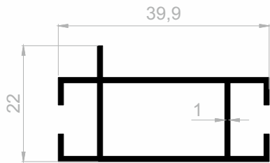
J 1964 DISPLAY PROFILE GEWICHT : 0,354 kg/m
