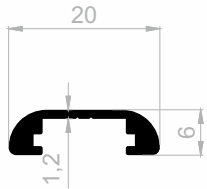
J 1509 DISPLAY PROFILE GEWICHT : 0,140 kg/m
