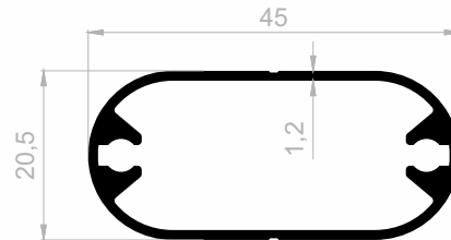
J 1056 DISPLAY PROFILE GEWICHT : 0,490 kg/m
