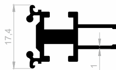
J 1161 DISPLAY PROFILE GEWICHT : 0,330 kg/m
