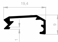
J 1180 DISPLAY PROFILE GEWICHT : 0,108 kg/m
