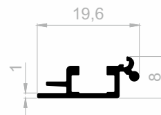
J 1161 DISPLAY PROFILE GEWICHT : 0,330 kg/m
