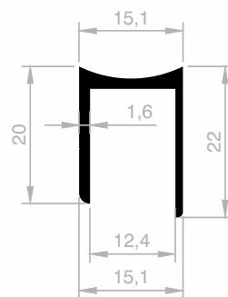
JM 4498 WC PROFILE GEWICHT : 0,216 kg/m
