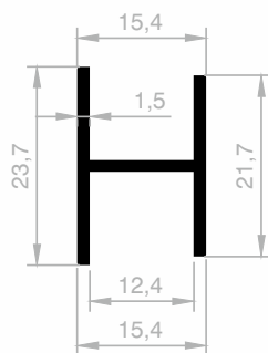
JM 4634 WC PROFILE GEWICHT : 0,236 kg/m
