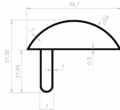
JM 6407 WC PROFILE GEWICHT : 0,399 kg/m
