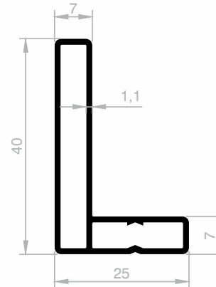
JM 5858 WC PROFILE GEWICHT : 0,387 kg/m
