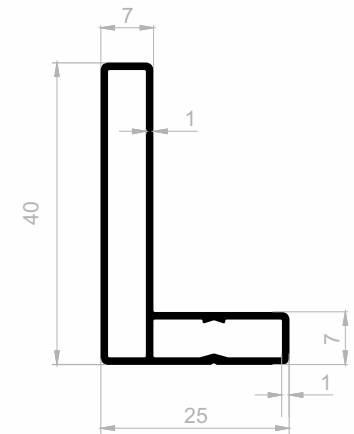
JM 6410 WC PROFILE GEWICHT : 0,357 kg/m
