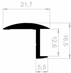
JM 6408 WC PROFILE GEWICHT : 0,198 kg/m
