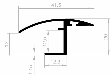
JM 4637 WC PROFILE GEWICHT : 0,308 kg/m
