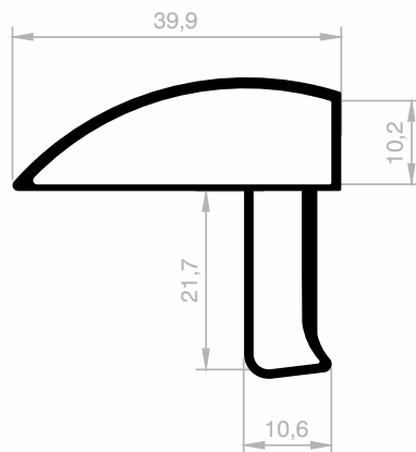
JM 6209 WC PROFILE GEWICHT : 0,478 kg/m
