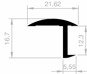
JM 4638 WC PROFILE GEWICHT : 0,202 kg/m
