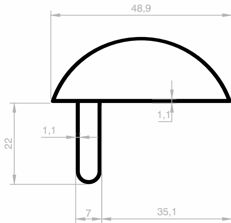
JM 4636 WC PROFILE GEWICHT : 0,464 kg/m
