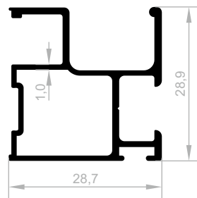
JM 1975 SEITLICHER GRIFF STANDARD GEWICHT : 0,420 kg/m
