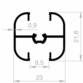
JM 6240 MITTENVERBINDER GEWICHT : 0,249 kg/m
