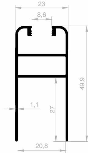
JM 1040 BODENVERBINDER GEWICHT : 0,468 kg/m
