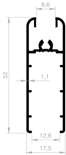
JM 4607 BODENVERBINDER GEWICHT : 0,451 kg/m
