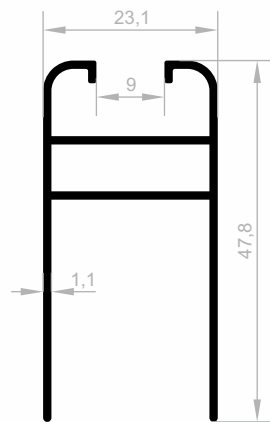
JM 1598 BODENVERBINDER GEWICHT : 0,447 kg/m
