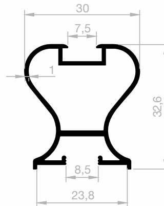
JM 6248 ECONOMIC GRIFF GEWICHT : 0,379 kg/m
