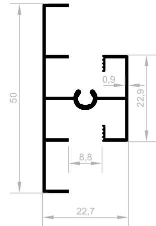
JM 1552 MITTENVERBINDER GEWICHT : 0,360 kg/m
