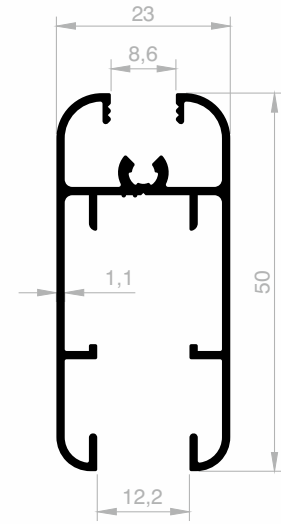
JM 6226 BODENVERBINDER GEWICHT : 0,534 kg/m
