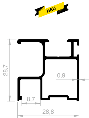
JM 1588 SEITLICHER GRIFF STANDARD GEWICHT : 0,420 kg/m
