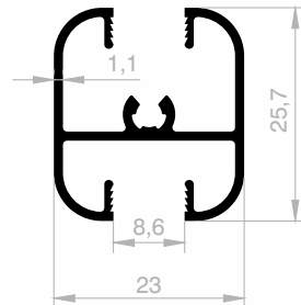
JM 1002 MITTENVERBINDER GEWICHT : 0,335 kg/m
