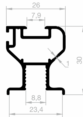
JM 1076 ECONOMIC GRIFF GEWICHT : 0,365 kg/m
