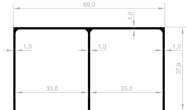
JM 1038 DECKENSCHIENE GEWICHT : 0,496 kg/m
