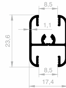
JM 4610 MITTENVERBINDER GEWICHT : 0,270 kg/m
