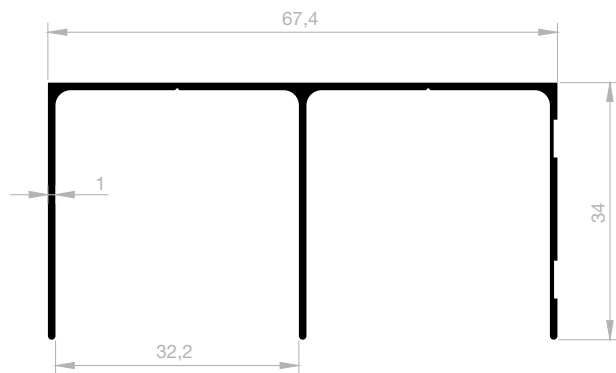
JM 5829 DECKENSCHIENE GEWICHT : 0,447 kg/m
