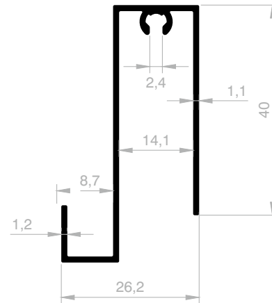
JM 4555 OBERE / UNTERE VERBINDER GEWICHT : 0,419 kg/m
