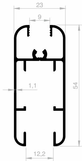
JM 3539 BODENVERBINDER GEWICHT : 0,570 kg/m
