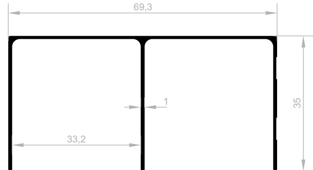
JM 1219-A DECKENSCHIENE GEWICHT : 0,429 kg/m
