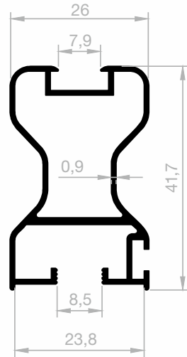
JM 6235 BREIT GRIFF GEWICHT : 0,443 kg/m
