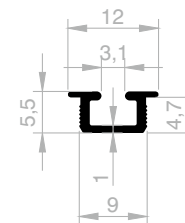
JM 1583 EINGebaUTE BODEN/DECKENSCHIENE GEWICHT : 0,073 kg/m
