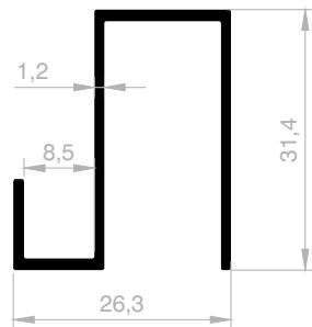
JM 1584 OBERE / UNTERE VERBINDER GEWICHT : 0,334 kg/m
