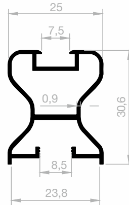
JM 6236 ECONOMIC GRIFF GEWICHT : 0,340 kg/m
