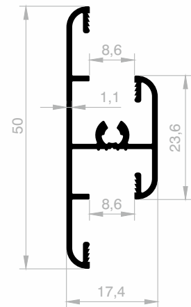
JM 4608 MITTENVERBINDER GEWICHT : 0,354 kg/m
