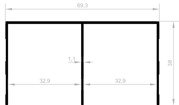
JM 1597 DECKENSCHIENE GEWICHT : 0,553 kg/m
