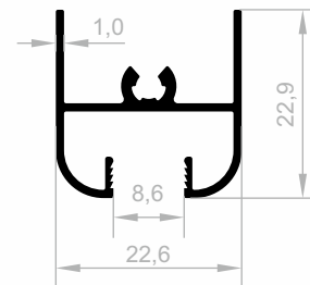
JM 1037 DECKENVERBINDER GEWICHT : 0,259 kg/m
