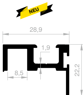
JM 1586 CHMALSEITIGER GRIFF GEWICHT : 0,417 kg/m
