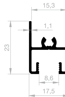
JM 3545 DECKENVERBINDER GEWICHT : 0,265 kg/m
