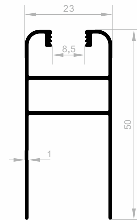
JM 1230 BODENVERBINDER GEWICHT : 0,440 kg/m
