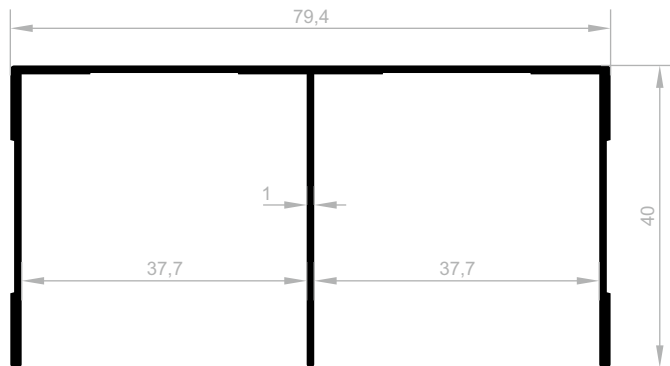
JM 1734 DECKENSCHIENE GEWICHT : 0,599 kg/m
