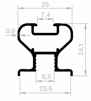
JM 6260 ECONOMIC GRIFF GEWICHT : 0,295 kg/m
