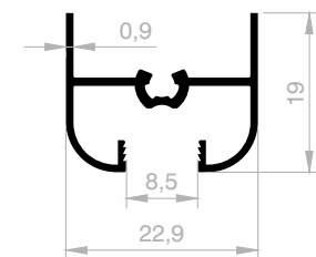
JM 6241 DECKENVERBINDER GEWICHT : 0,205 kg/m
