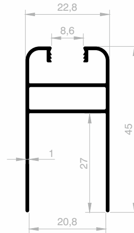
JM 6225 BODENVERBINDER GEWICHT : 0,402 kg/m
