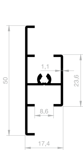
JM 3543 MITTENVERBINDER GEWICHT : 0,355 kg/m
