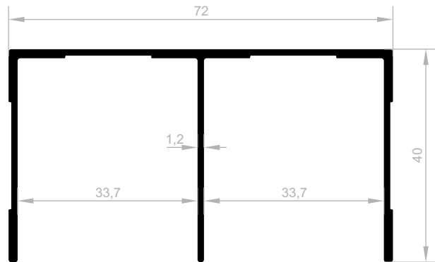
JM 1564 DECKENSCHIENE GEWICHT : 0,710 kg/m
