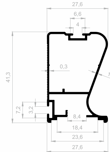
JM 10065 GRIFF GEWICHT : 0,447 kg/m
