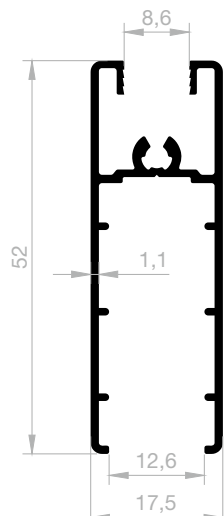
JM 3542 BODENVERBINDER GEWICHT : 0,454 kg/m
