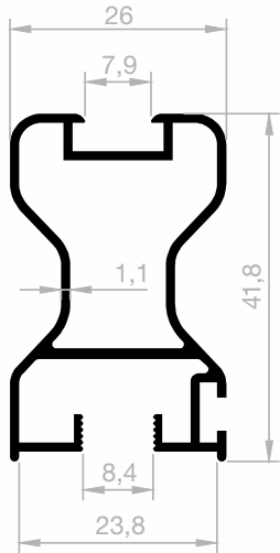
JM 1035 BREIT GRIFF GEWICHT : 0,508 kg/m
