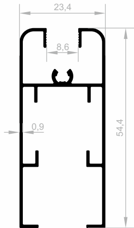
JM 8268 BODENVERBINDER GEWICHT : 0,471 kg/m
