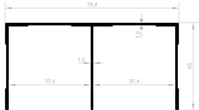
JM 1569 DECKENSCHIENE GEWICHT : 0,734 kg/m
