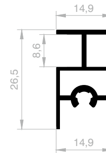
JM 1585 MITTENVERBINDER GEWICHT : 0,308 kg/m
