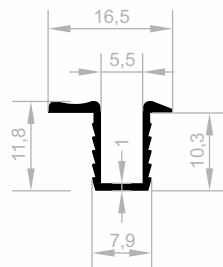
JM 1900 BODENSCHIENE GEWICHT : 0,113 kg/m
