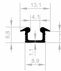
JM 5860 EINGEBAUT UNTER OBER SCHIENE GEWICHT : 0,082 kg/m
