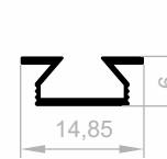
JM 2229 UNTER OBER DECKENSCHIENE GEWICHT : 0,073 kg/m
