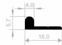
JM 1969 BODENSCHIENE GEWICHT : 0,100 kg/m
