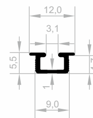
JM 1583 EINGEBAUT UNTER OBER SCHIENE GEWICHT : 0,073 kg/m
