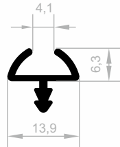
JM 3821 UNTER ASCHIENE GEWICHT : 0,132 kg/m
