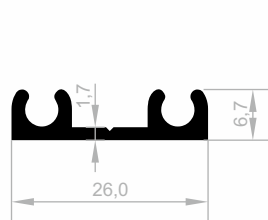
JM 1821 BODENSCHIENE GEWICHT : 0,222 kg/m
