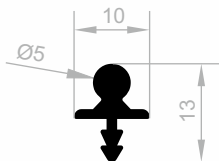
JM 2638 SINGLE BODENSCHIENE GEWICHT : 0,130 kg/m
