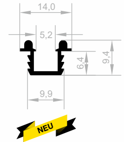
JM 10030 UNTER ASCHIENE GEWICHT : 0,108 kg/m
