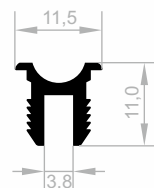
JM 1901 BODENSCHIENE GEWICHT : 0,134 kg/m
