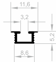
JM 3474 EINGEBAUT UNTER OBER SCHIENE GEWICHT : 0,054 kg/m
