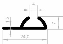
JM 1756 UNTER ASCHIENE GEWICHT : 0,152 kg/m
