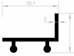
JM 1820 TRAGER DECKENSCHIENE GEWICHT : 0,325 kg/m
