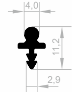
JM 1100 SINGLE BODENSCHIENE GEWICHT : 0,100 kg/m
