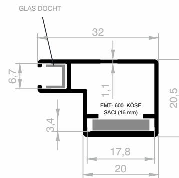
JM 4752 RAHMEN ABDECKUNG GEWICHT : 0,346 kg/m
