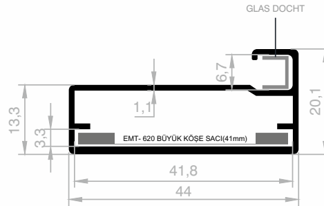
JM 1212 RAHMEN ABDECKUNG GEWICHT : 0,437 kg/m
