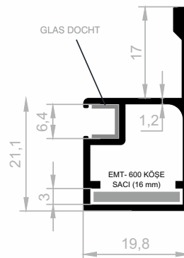
JM 4649 RAHMEN ABDECKUNG GEWICHT : 0,383 kg/m
