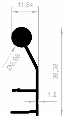
JM 2005 RAHMEN ABDECKUNG GEWICHT : 0,347 kg/m
