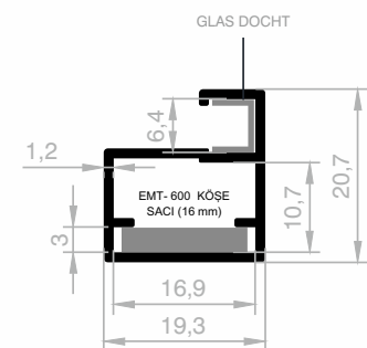
JM 3931 RAHMEN ABDECKUNG GEWICHT : 0,267 kg/m
