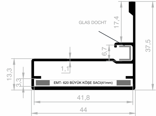
JM 4646 RAHMEN ABDECKUNG GEWICHT : 0,516 kg/m
