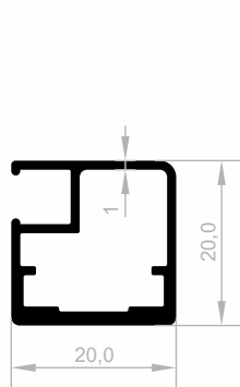
JM 3385 RAHMEN ABDECKUNG GEWICHT : 0,312 kg/m
