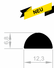
JM 8900 MOBEL GRIFF PROFILE GEWICHT : 0,176 kg/m
