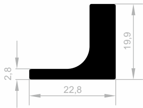
JM 1868 MOBEL GRIFF PROFILE GEWICHT : 0,512 kg/m
