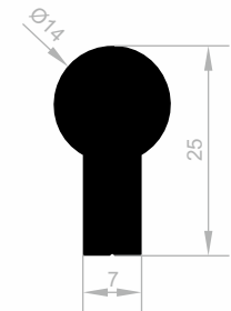
JM 1965 MOBEL GRIFF PROFILE GEWICHT : 0,632 kg/m
