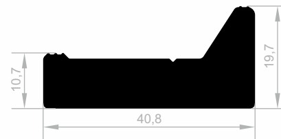
JM 1961 MOBEL GRIFF PROFILE GEWICHT : 1,255 kg/m
