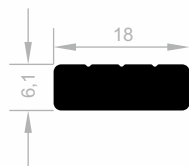
JM 8151 MOBEL GRIFF PROFILE GEWICHT : 0,293 kg/m
