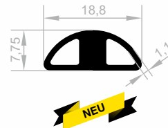
JM 8396 MOBEL GRIFF PROFILE GEWICHT : 0,201 kg/m
