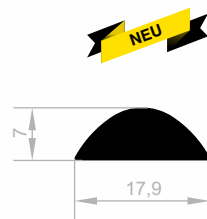
JM 8899 MOBEL GRIFF PROFILE GEWICHT : 0,238 kg/m
