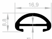
JM 1149 MOBEL GRIFF PROFILE GEWICHT : 0,152 kg/m
