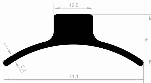
JM 2000 MOBEL GRIFF PROFILE GEWICHT : 1,339 kg/m
