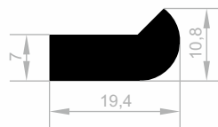
JM 2007 MOBEL GRIFF PROFILE GEWICHT : 0,379 kg/m
