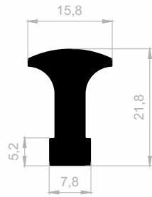
JM 10078 MOBEL GRIFF PROFILE GEWICHT : 0,466 kg/m
