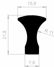
JM 6406 MOBEL GRIFF PROFILE GEWICHT : 0,491 kg/m
