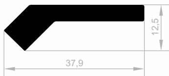
JM 1514 MOBEL GRIFF PROFILE GEWICHT : 0,566 kg/m
