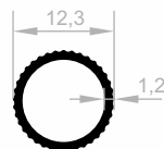
JM 1166 MOBEL GRIFF PROFILE GEWICHT : 0,103 kg/m
