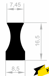
JM 8921 MOBEL GRIFF PROFILE GEWICHT : 0,277 kg/m
