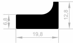
JM 1776 MOBEL GRIFF PROFILE GEWICHT : 0,422 kg/m
