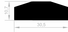
JM 2009 MOBEL GRIFF PROFILE GEWICHT : 0,797 kg/m
