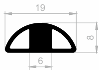
JM 6394 MOBEL GRIFF PROFILE GEWICHT : 0,218 kg/m
