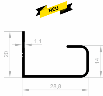
JM 8729 MOBEL GRIFF PROFILE GEWICHT : 0,198 kg/m
