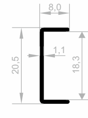
JM 2979 KANTENABDECKUNGS GEWICHT : 0,100 kg/m
