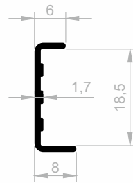
JM 1089 KANTENABDECKUNGS GEWICHT : 0,115 kg/m
