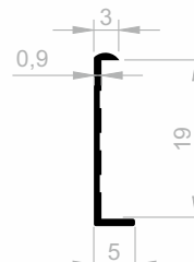
JM 6232 KANTENABDECKUNGS GEWICHT : 0,062 kg/m
