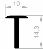
JM 5756 KANTENABDECKUNGS GEWICHT : 0,101 kg/m
