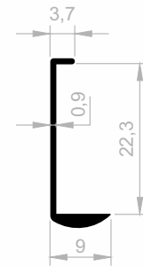
JM 6231 KANTENABDECKUNGS GEWICHT : 0,101 kg/m
