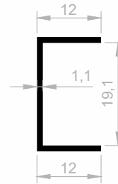
JM 4624 KANTENABDECKUNGS GEWICHT : 0,129 kg/m
