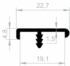
JM 1091 KANTENABDECKUNGS GEWICHT : 0,105 kg/m
