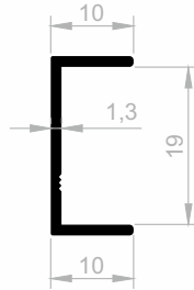
JM 4598 KANTENABDECKUNGS GEWICHT : 0,140 kg/m
