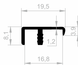
JM 1067 KANTENABDECKUNGS GEWICHT : 0,145 kg/m
