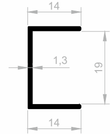
JM 4514 KANTENABDECKUNGS GEWICHT : 0,169 kg/m
