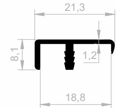
JM 1070 KANTENABDECKUNGS GEWICHT : 0,150 kg/m
