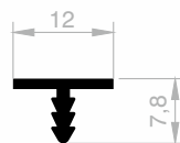
JM 1067 KANTENABDECKUNGS GEWICHT : 0,145 kg/m
