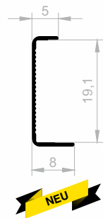
JM 6245 KANTENABDECKUNGS GEWICHT : 0,063 kg/m
