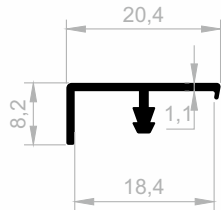
JM 1091 KANTENABDECKUNGS GEWICHT : 0,105 kg/m
