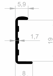
JM 4581 KANTENABDECKUNGS GEWICHT : 0,112 kg/m
