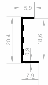
JM 1926 KANTENABDECKUNGS GEWICHT : 0,087 kg/m
