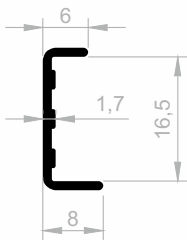
JM 1781 KANTENABDECKUNGS GEWICHT : 0,090 kg/m
