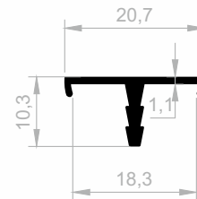
JM 6231 KANTENABDECKUNGS GEWICHT : 0,101 kg/m
