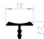
JM 4656 KANTENABDECKUNGS GEWICHT : 0,170 kg/m
