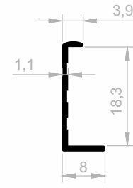
JM 5698 KANTENABDECKUNGS GEWICHT : 0,085 kg/m
