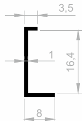
JM 1113 KANTENABDECKUNGS GEWICHT : 0,080 kg/m
