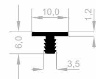
JM 4653 KANTENABDECKUNGS GEWICHT : 0,199 kg/m
