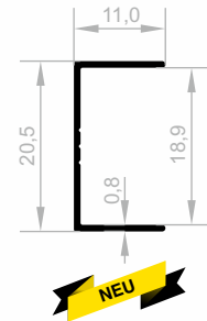
JM 8531 KANTENABDECKUNGS GEWICHT : 0,088 kg/m
