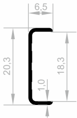
JM 3475 KANTENABDECKUNGS GEWICHT : 0,067 kg/m
