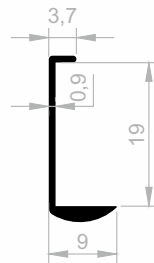
JM 6233 KANTENABDECKUNGS GEWICHT : 0,093 kg/m
