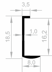
JM 8531 KANTENABDECKUNGS GEWICHT : 0,088 kg/m
