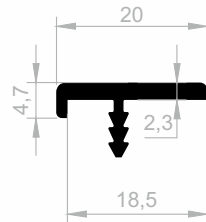
JM 4324 KANTENABDECKUNGS GEWICHT : 0,175 kg/m
