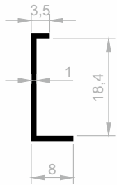
JM 1146 KANTENABDECKUNGS GEWICHT : 0,085 kg/m
