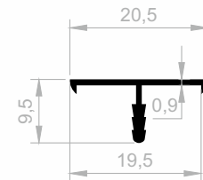
JM 1123 KANTENABDECKUNGS GEWICHT : 0,075 kg/m
