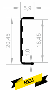
JM 8547 KANTENABDECKUNGS GEWICHT : 0,069 kg/m
