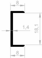
JM 1507 KANTENABDECKUNGS GEWICHT : 0,135 kg/m
