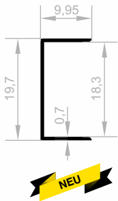
JM 8727 KANTENABDECKUNGS GEWICHT : 0,072 kg/m
