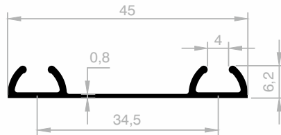
JM 5941 BODENSCHIENE GEWICHT : 0,200 kg/m
