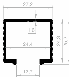
JM 4098 DECKENSCHIENE GEWICHT : 0,355 kg/m
