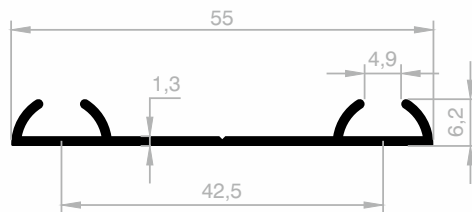
JM 4095 BODENSCHIENE GEWICHT : 0,280 kg/m
