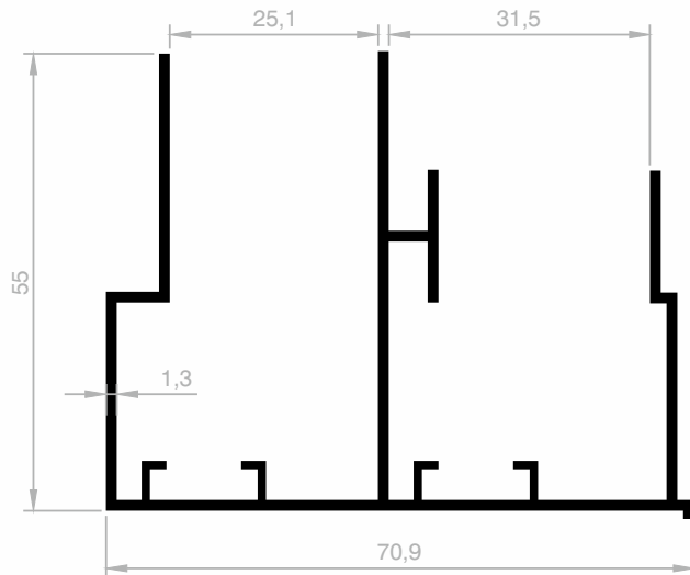
JM 4611 OBERE HÄNGESCHIENE GEWICHT : 0,949 kg/m
