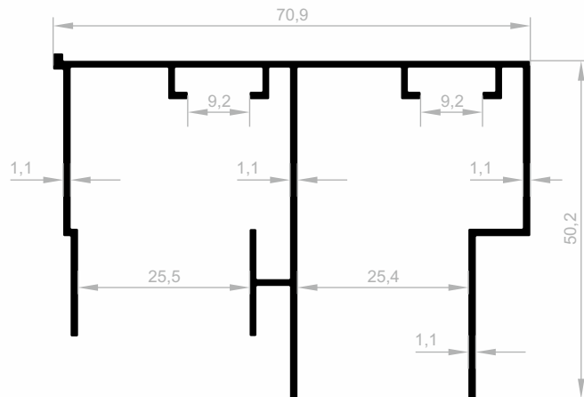
JM 8203 DECKENSCHIENE GEWICHT : 0,767 kg/m
