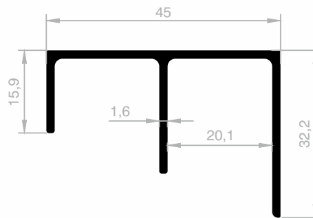
JM 3618 BODENSCHIENE GEWICHT : 0,494 kg/m
