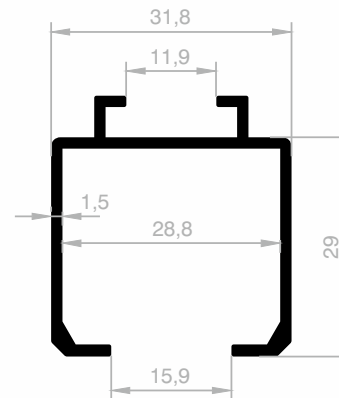
JM 1090 OBERE TÜRSCHIENE GEWICHT : 0,470 kg/m
