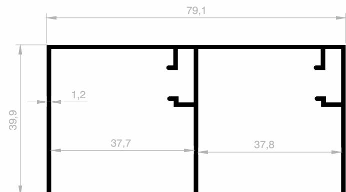
JM 6199 DECKENSCHIENE GEWICHT : 0,706 kg/m
