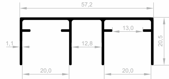
JM 1604 DECKENSCHIENE GEWICHT : 0,445 kg/m
