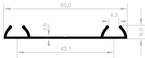
JM 1605 BODENSCHIENE GEWICHT : 0,225 kg/m
