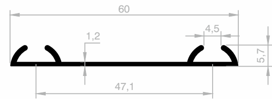
JM 1195 BODENSCHIENE GEWICHT : 0,265 kg/m
