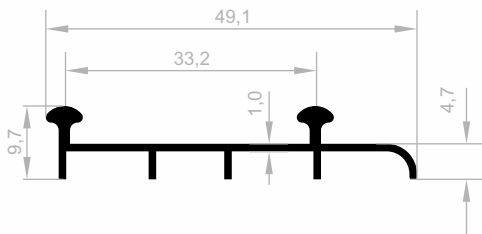
JM 1596 DECKENSCHIENE GEWICHT : 0,247 kg/m
