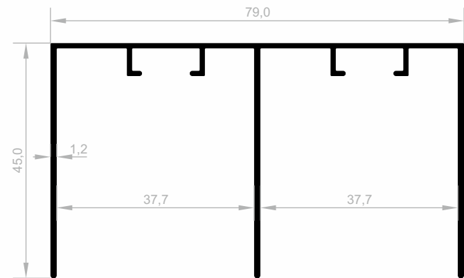
JM 8202 DECKENSCHIENE GEWICHT : 0,653 kg/m
