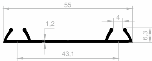
JM 1731 BODENSCHIENE GEWICHT : 0,225 kg/m
