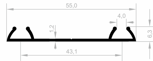
JM 1782 BODENSCHIENE GEWICHT : 0,255 kg/m
