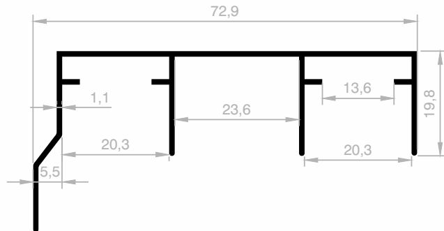
JM 4031 DECKENSCHIENE GEWICHT : 0,491 kg/m
