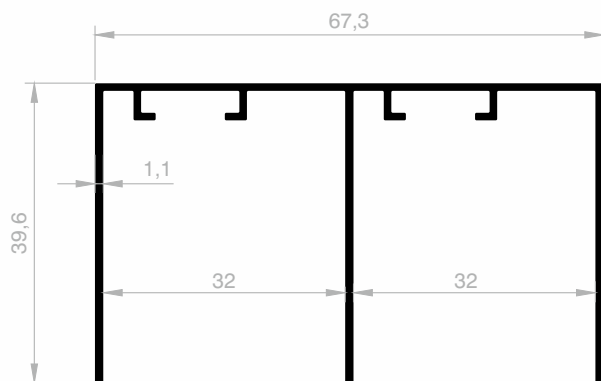
JM 5640 DECKENSCHIENE GEWICHT : 0,591 kg/m
