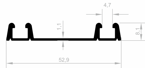
JM 10032 BODENSCHIENE GEWICHT : 0,339 kg/m
