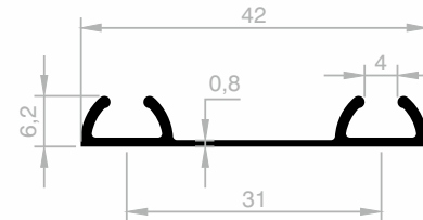
JM 5940 BODENSCHIENE GEWICHT : 0,193 kg/m
