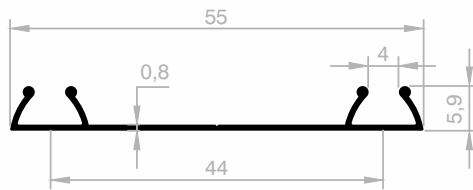
JM 4898 BODENSCHIENE GEWICHT : 0,175 kg/m
