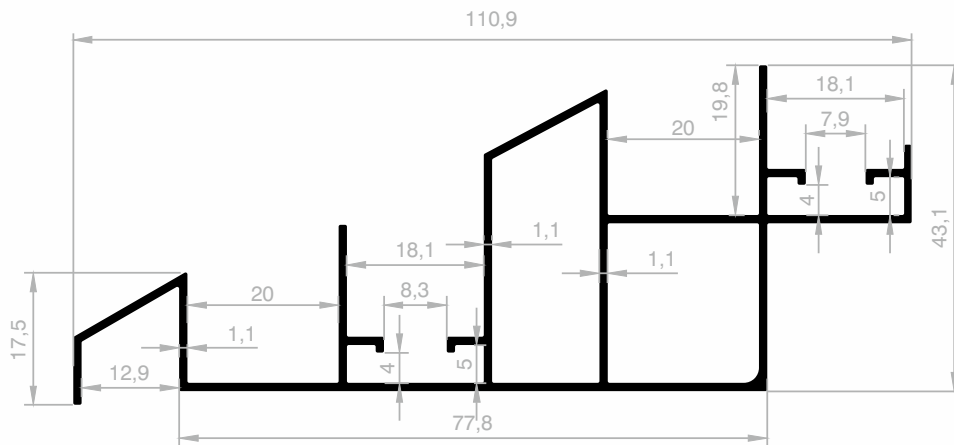
JM 4503 OBERE HÄNGESCHIENE GEWICHT : 1,010 kg/m
