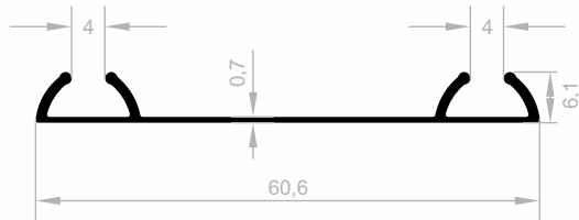
JM 3472 BODENSCHIENE GEWICHT : 0,200 kg/m
