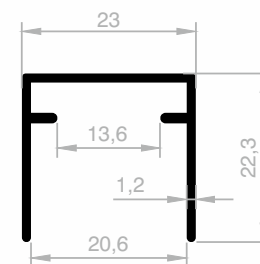
JM 2064 DECKENSCHIENE GEWICHT : 0,230 kg/m
