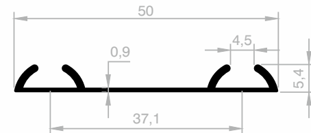
JM 4029 BODENSCHIENE GEWICHT : 0,230 kg/m
