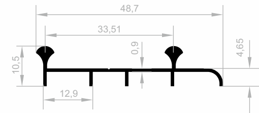
JM 1220 DECKENSCHIENE GEWICHT : 0,233 kg/m
