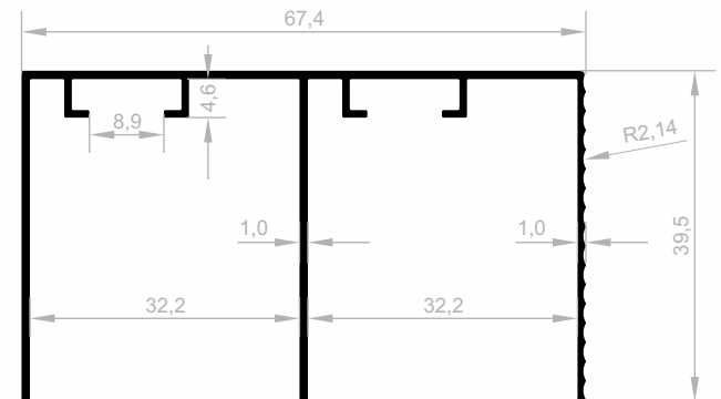
JM 8602 DECKENSCHIENE GEWICHT : 0,539 kg/m
