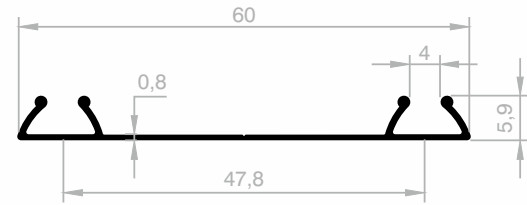
JM 4897 BODENSCHIENE GEWICHT : 0,189 kg/m
