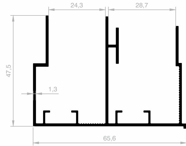
JM 4833 OBERE HÄNGESCHIENE GEWICHT : 0,835 kg/m
