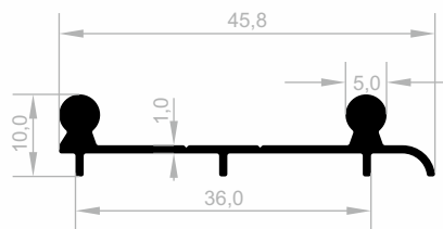
JM 1714 DECKENSCHIENE GEWICHT : 0,285 kg/m
