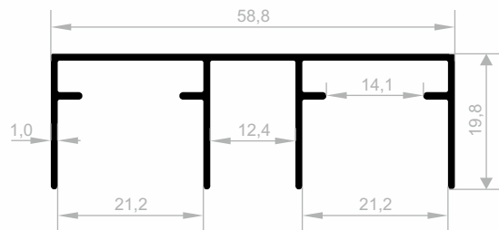
JM 1711 DECKENSCHIENE GEWICHT : 0,404 kg/m
