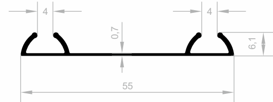
JM 3473 BODENSCHIENE GEWICHT : 0,189 kg/m
