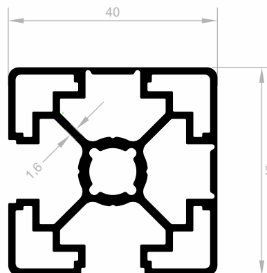
J 10099 SIGMA PROFILE GEWICHT : 1,218 kg/m
