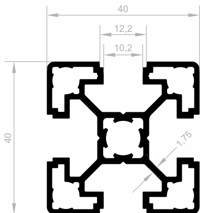
J 10097 SIGMA PROFILE GEWICHT : 1,215 kg/m
