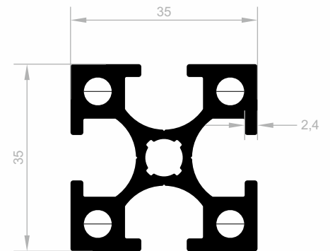
J 1590 SIGMA PROFILE GEWICHT : 1,375 kg/m
