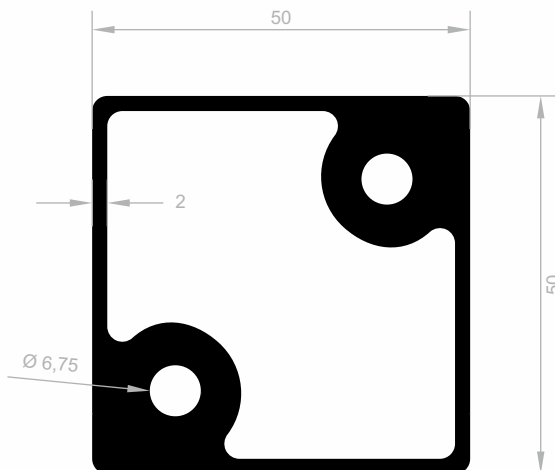
J 1627 SIGMA PROFILE GEWICHT : 2,385 kg/m
