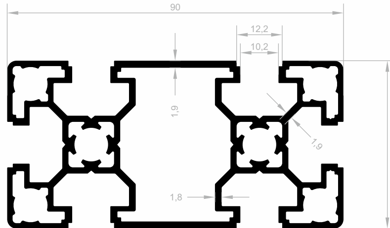
J 10141 SIGMA PROFILE GEWICHT : 2,567 kg/m
