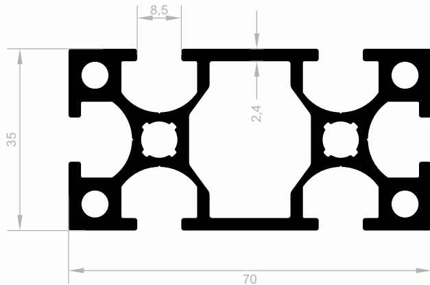
J 1591 SIGMA PROFILE GEWICHT : 2,182 kg/m
