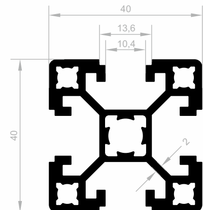
J 6662 SIGMA PROFILE GEWICHT : 1,534 kg/m
