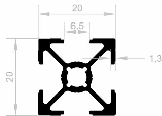
J 2392 SIGMA PROFILE GEWICHT : 0,360 kg/m
