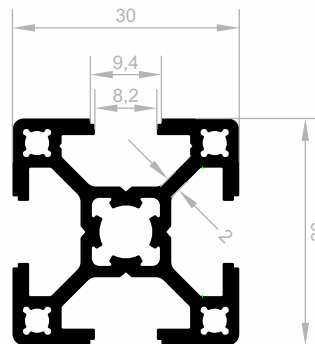
J 10144 SIGMA PROFILE GEWICHT : 0,856 kg/m
