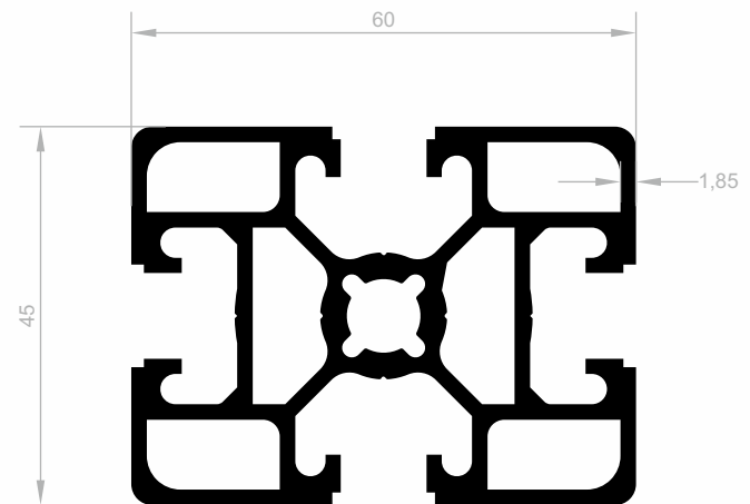
J 2168 SIGMA PROFILE GEWICHT : 2,333 kg/m
