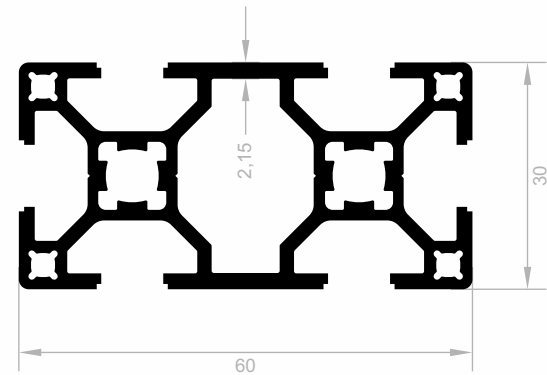
J 6096 SIGMA PROFILE GEWICHT : 1,453 kg/m
