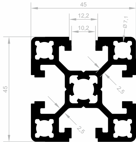
J 10143 SIGMA PROFILE GEWICHT : 2,066 kg/m
