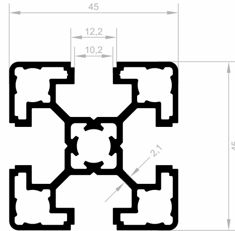
J 6688 SIGMA PROFILE GEWICHT : 1,523 kg/m
