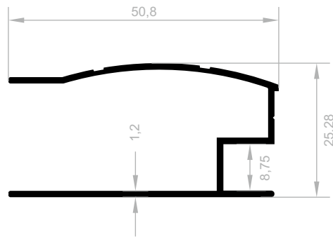
J 10164 DUSCH-KABINETT PROFILE (KAMELYA SERIE) GEWICHT : 0,427 kg/m
