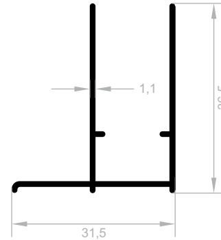
J 1250 DUSCH-KABINETT PROFILE (BELLA SERIE) GEWICHT : 0,319 kg/m
