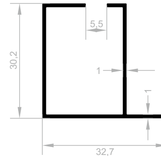
J 6594 DUSCH-KABINETT PROFILE (PRATIKO SERIE) GEWICHT : 0,287 kg/m
