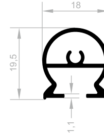
J 1252 DUSCH-KABINETT PROFILE (BELLA SERIE) GEWICHT : 0,254 kg/m
