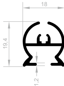
J 1258 DUSCH-KABINETT PROFILE (BELLA SERIE) GEWICHT : 0,267 kg/m
