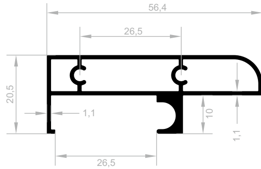
J 6596 DUSCH-KABINETT PROFILE (KAMELYA SERIE) GEWICHT : 0,593 kg/m
