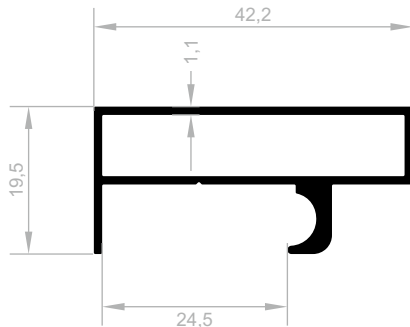
J 6595 DUSCH-KABINETT PROFILE (PRATIKO SERIE) GEWICHT : 0,407 kg/m
