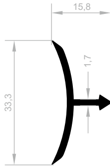
J 1091 DUSCH-KABINETT PROFILE (BELLA SERIE) GEWICHT : 0,217 kg/m
