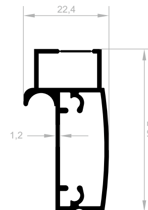
J 1873 DUSCH-KABINETT PROFILE (BELLA SERIE) GEWICHT : 0,492 kg/m
