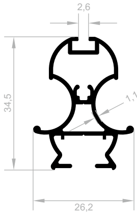
J 1257 DUSCH-KABINETT PROFILE (BELLA SERIE) GEWICHT : 0,443 kg/m
