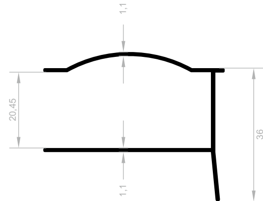
J 10216 DUSCH-KABINETT PROFILE (RELAX SERIE) GEWICHT : 0,401 kg/m
