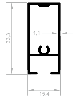
J 1256 DUSCH-KABINETT PROFILE (BELLA SERIE) GEWICHT : 0,338 kg/m
