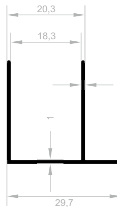
J 6597 DUSCH-KABINETT PROFILE (PRATIKO SERIE) GEWICHT : 0,220 kg/m
