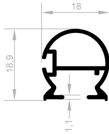
J 1251 DUSCH-KABINETT PROFILE (BELLA SERIE) GEWICHT : 0,240 kg/m
