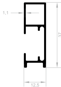
J 1253 DUSCH-KABINETT PROFILE (BELLA SERIE) GEWICHT : 0,308 kg/m
