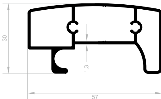
J 2087 DUSCH-KABINETT PROFILE (BELLA SERIE) GEWICHT : 0,797 kg/m
