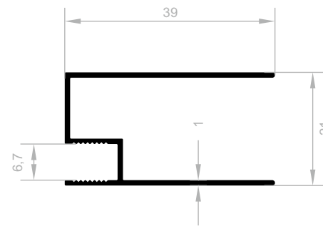
J 6593 DUSCH-KABINETT PROFILE (KAMELYA SERIE) GEWICHT : 0,284 kg/m
