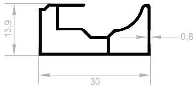
J 1110 DUSCH-KABINETT PROFILE (BELLA SERIE) GEWICHT : 0,230 kg/m
