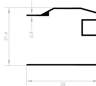
J 1106 DUSCH-KABINETT PROFILE (BELLA SERIE) GEWICHT : 0,282 kg/m
