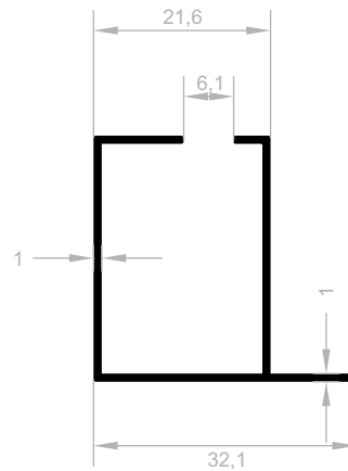
J 10345 DUSCH-KABINETT PROFILE GEWICHT : 0,280 kg/m
